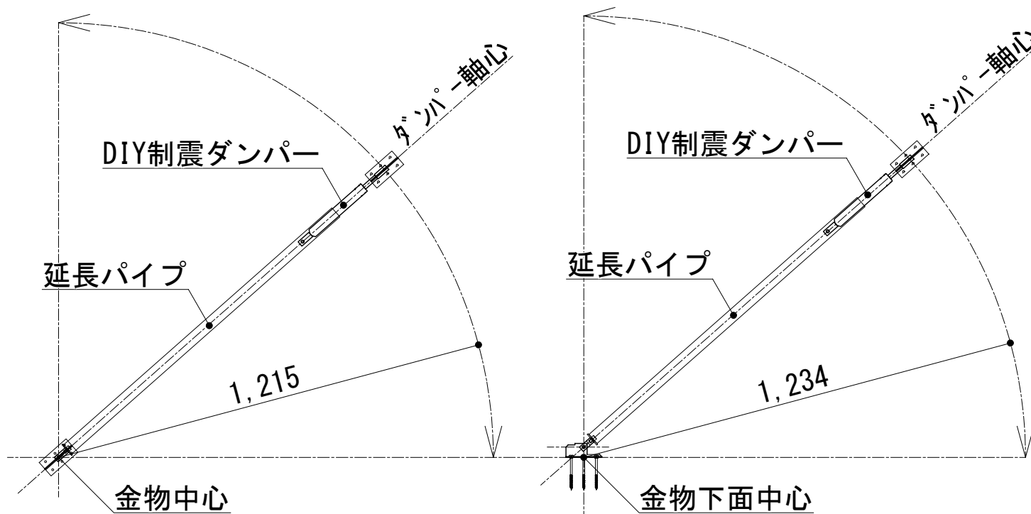
金物横-横 取付図
